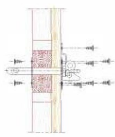
Seitenansicht / Schnitt ohne Pfosten
