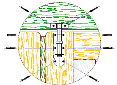
Feststellriegel oben
