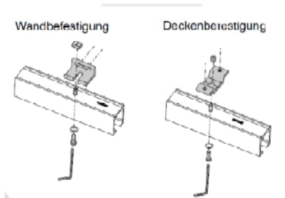
Wandbefestigung mit Befestigungswinkel Deckenbefestigung mit Deckenträger
