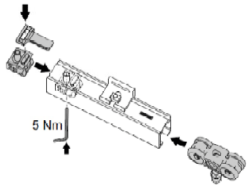
Rohrpuffer mit Feststellfeder Doppelrollwagen
