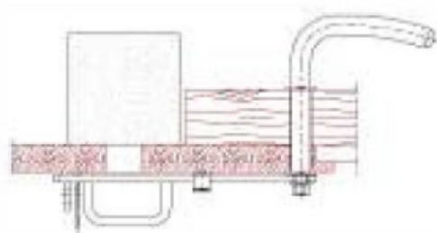
Draufsichten
