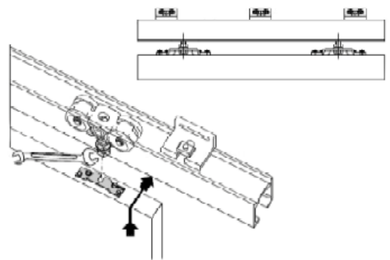
Aufhängeschraube
