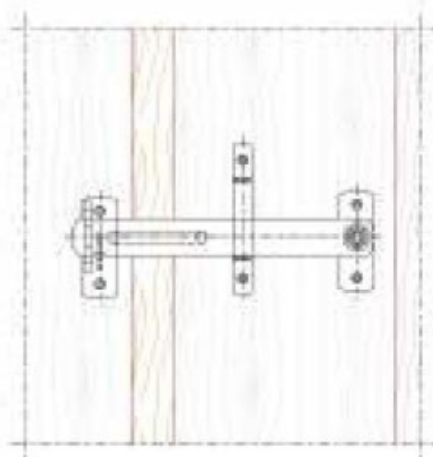
Vorderansicht
