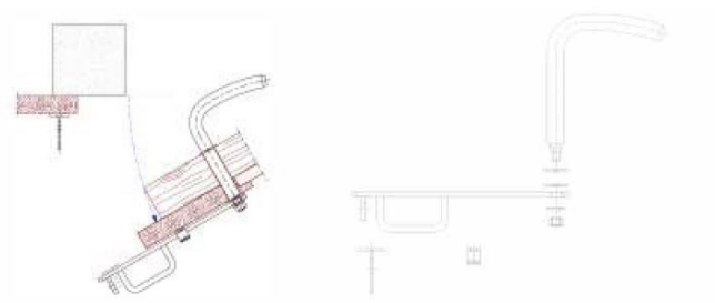
Seitenansicht / Schnitt ohne Pfosten
