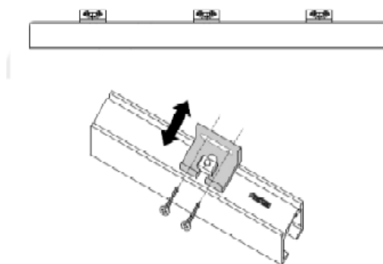
Wandbefestigung mit Befestigungswinkel
