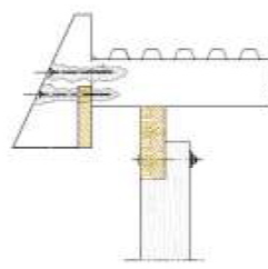
Befestigung des Pfannenreiters mit Torx-Schraube bis 8 x 240 mm Reiter vorbohren
